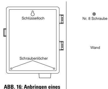
ABB. 16: Anbringen eines außeninstallierten Controllers
