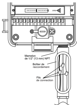
FIGURE 21 : Câblage à l'aide d'une boîte de raccordement
