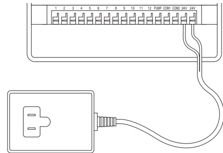
ABB. 17: Anschluß des Pumpenanlassers und des Hauptventils am Transformator
