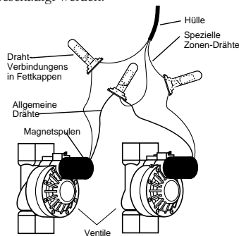
Abb. 22: Anschluß des Steuergerätekabels an den Ventilen
