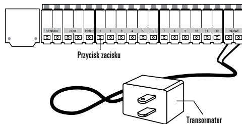
Rysunek 4: Podłączenie transformatora
