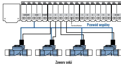
Rysunek 5: Podłączanie przewodu zraszacza
